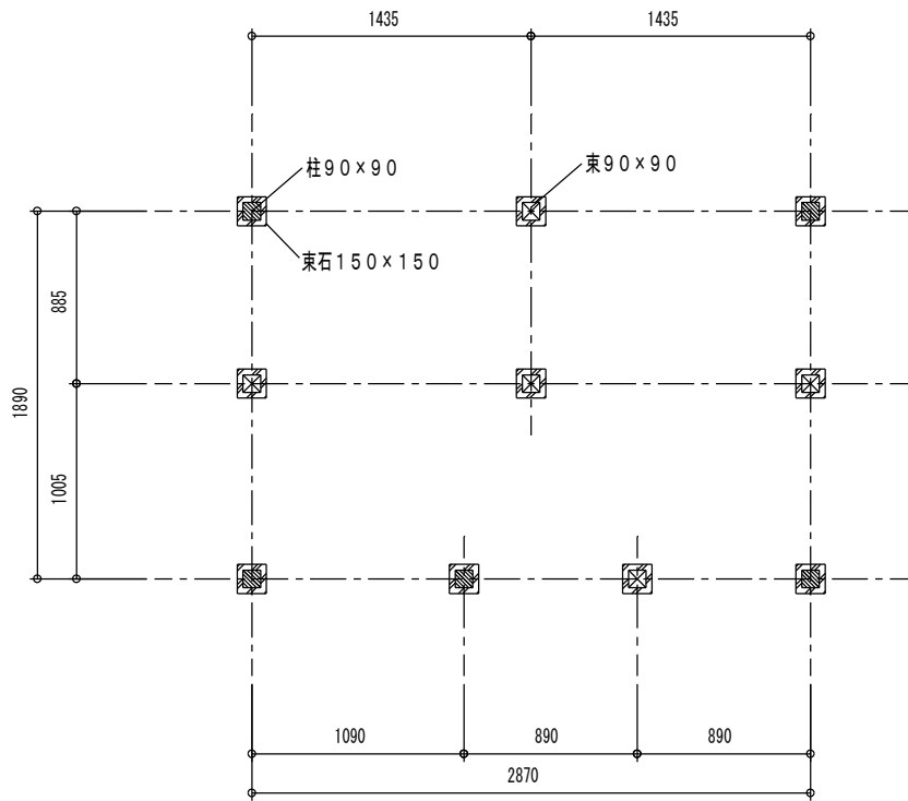
基礎・柱・束 伏せ図
