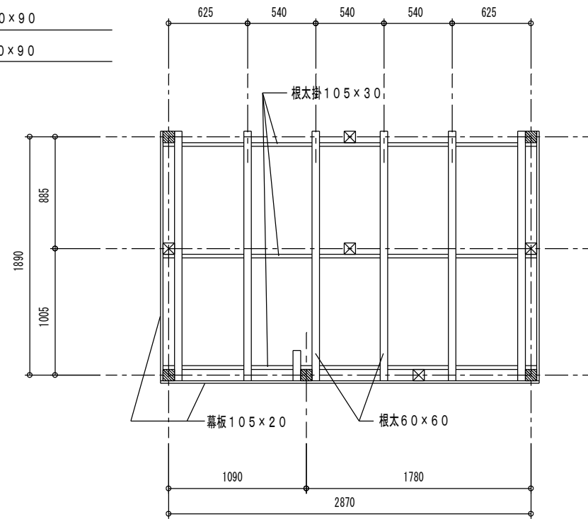
根太 伏せ図
