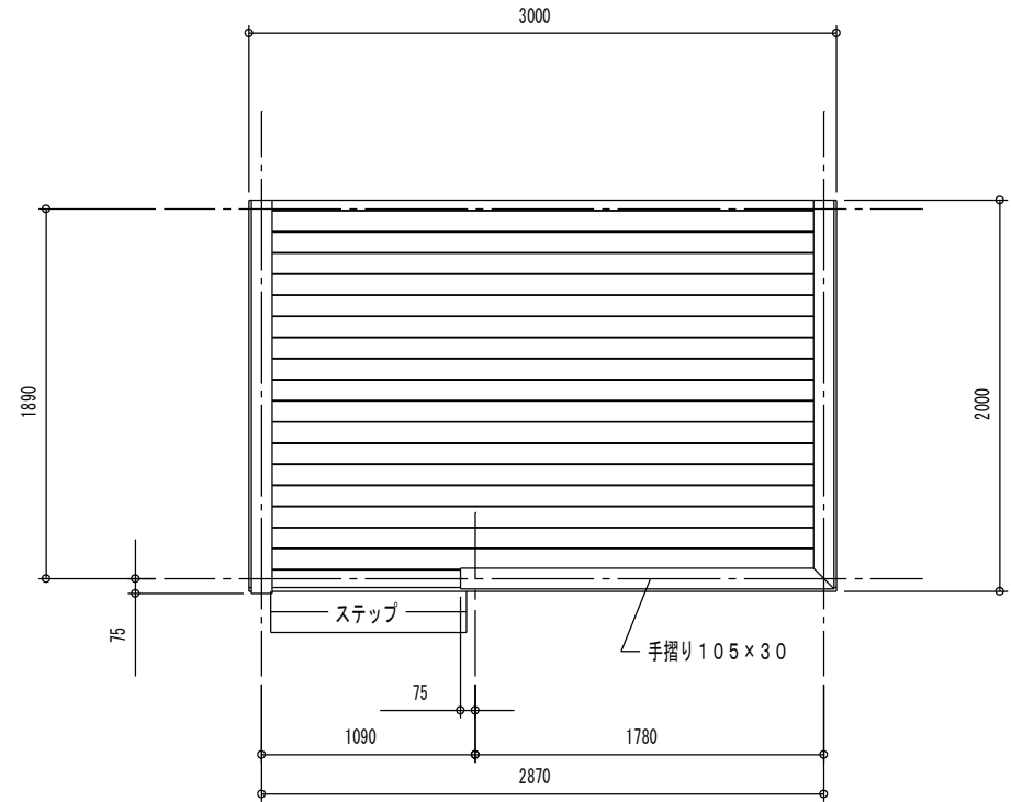
平面図
