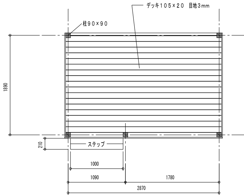
デッキ 伏せ図
