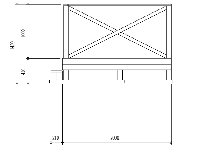
側面立面図
