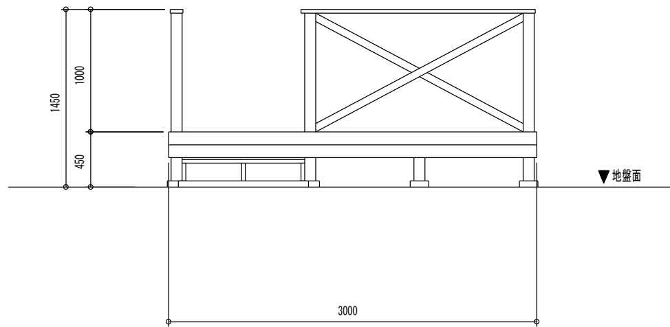
正面立面図
