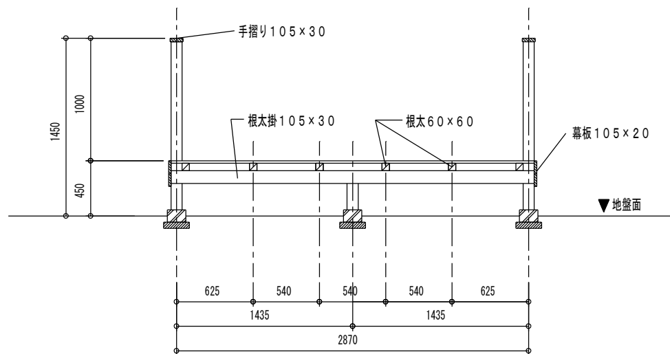
断面図
